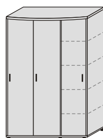
SG-43 150/65/200
